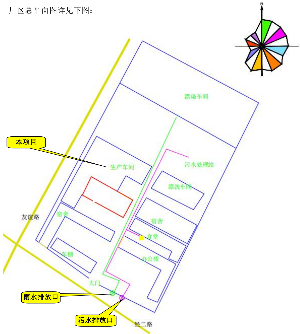
图 3.3-1 项目厂区总平面布置图
