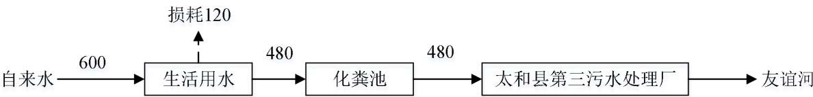
图 3.8-1 项目水量平衡图 (单位: t/d)
