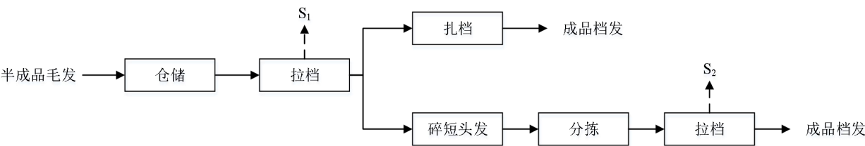
图 3.9-1 生产工艺生产工艺流程及产污节点图
